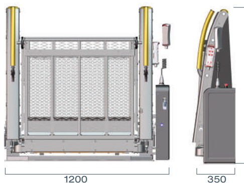
Typ AL1 Panorama 1200
